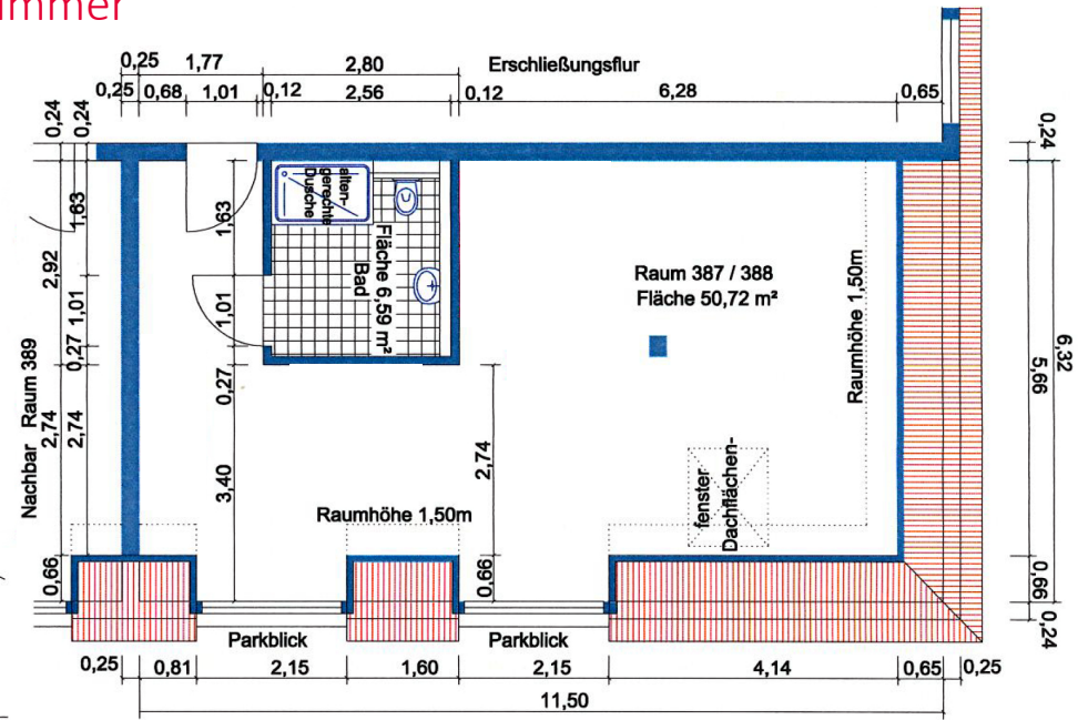
Lage Zimmer
